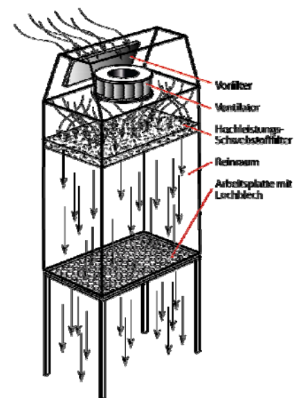
Funktionsskizze der asecos Laminar Flow Box
