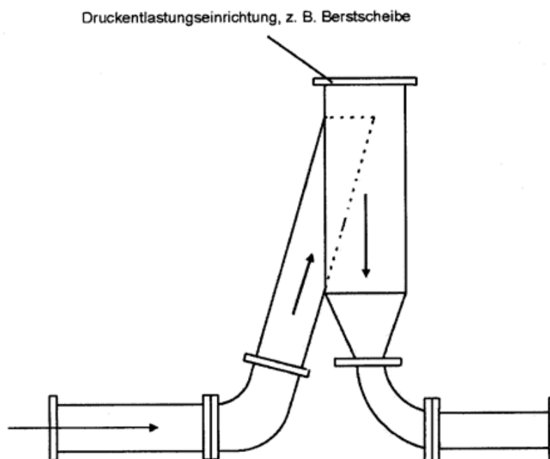
Bild 1: Schematische Darstellung eines Entlastungsschlotes
